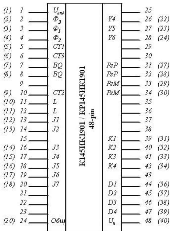
Рис.2 Расположение выводов микросхемы КР145ИК1901.
