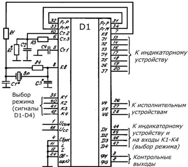
Типовая схема включения БИС К145ИК1901.
